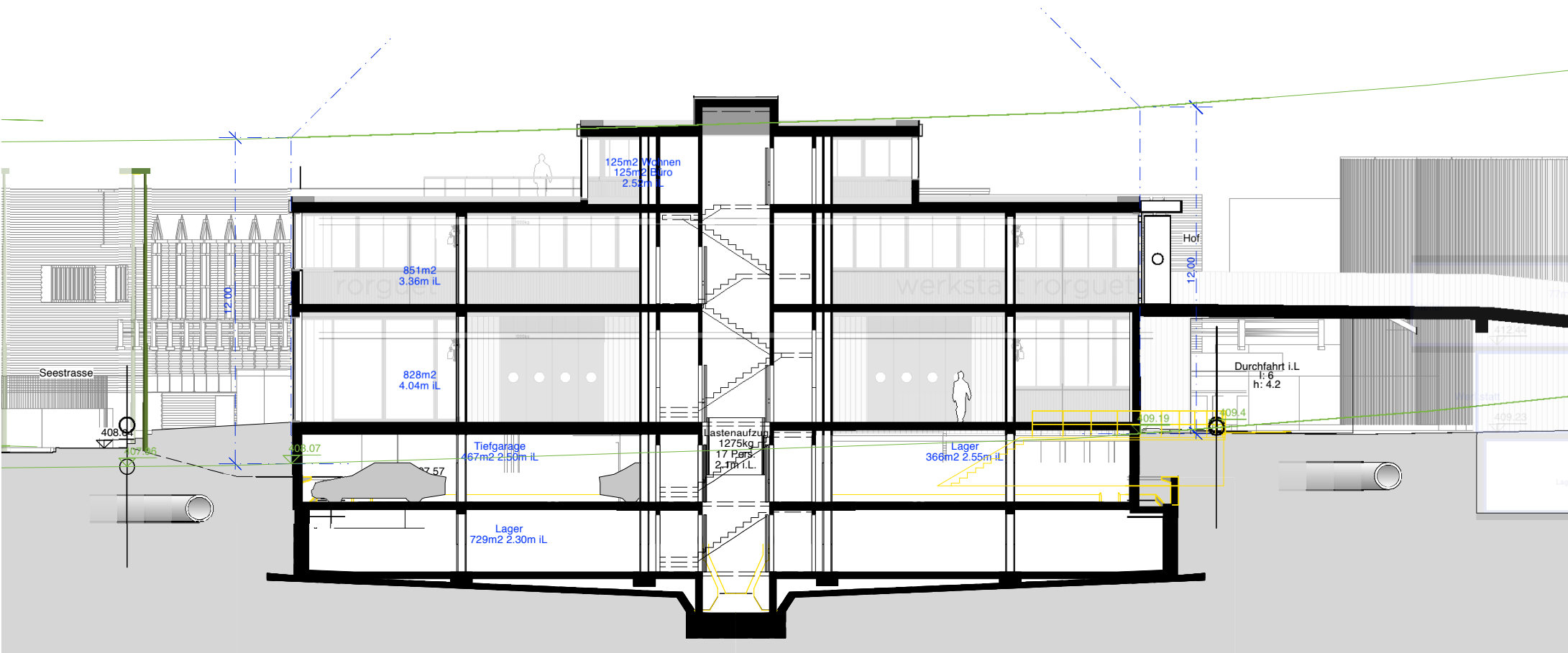
Schnitt quer
